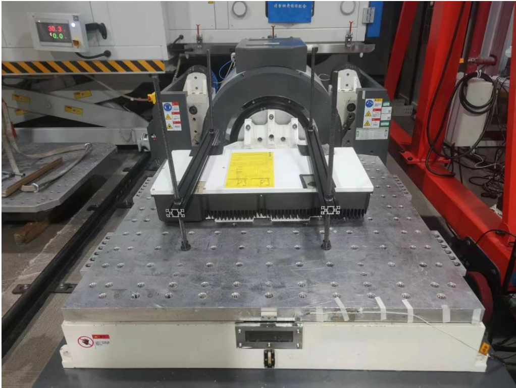
EUT-1 X 轴向随机振动（裸机）、正弦振动（裸机）固定照片
