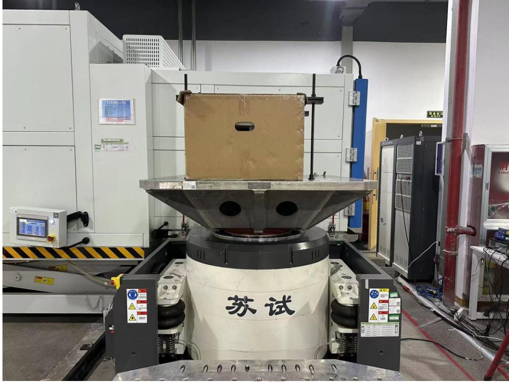
EUT-1 Z 轴向随机振动 (包装) 固定照片
