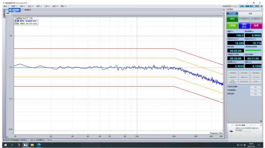
Y 轴向试验曲线
