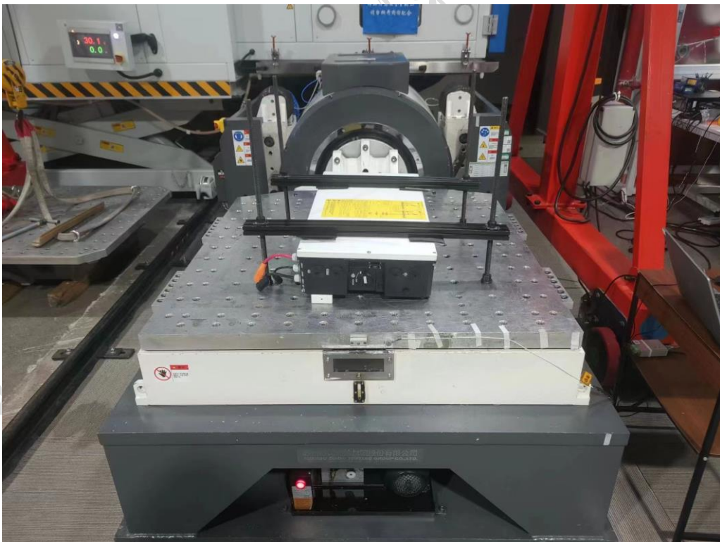
EUT-1 Y 轴向随机振动（裸机）、正弦振动（裸机）固定照片
