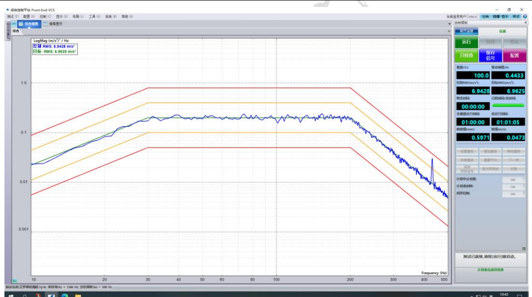
Z 轴向试验曲线
